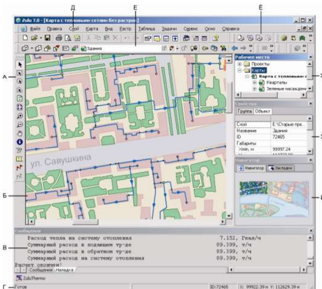
Рисунок 5.1. Общий вид системы Zulu. А - панель навигации по карте. Б - окно карты. В - окно сообщений. Г - строка состояния. Д – строка основного меню системы. Е – список загруженных в карту слоев. Ё – панель инструментов. Ж – окно проектов. З – окно свойств. И – окно навигации
