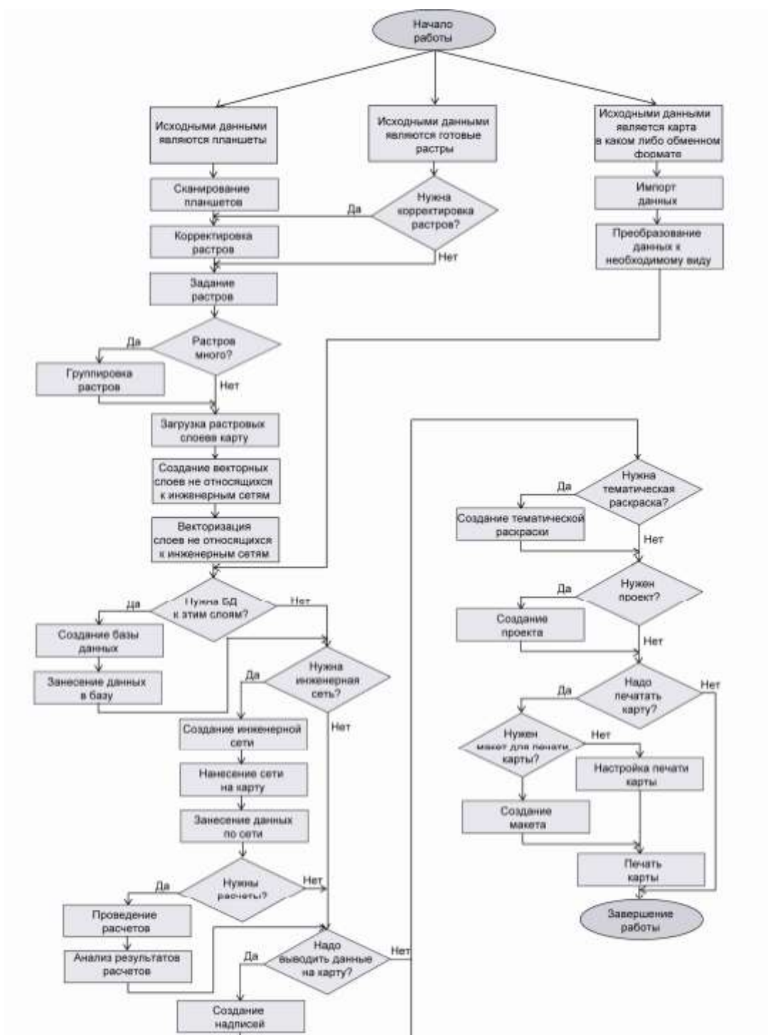
Рисунок 25.1. Алгоритм работы с системой
